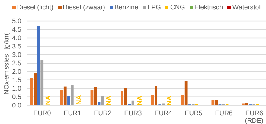
Figuur 5: Historisch verloop van NO x -emissies van bestelauto's op verschillende energiedragers.
